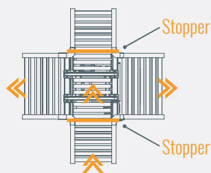
Haakse overgangseenheid, hoge capaciteit
